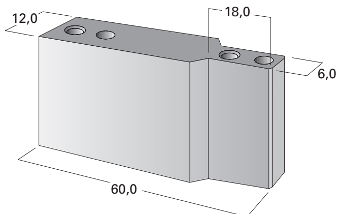
Sondergehäuse der Typenreihe LKV-12/VA Zur Realisierung kleiner Rastermaße, bevorzugt bei Kreis-Anordnung.
